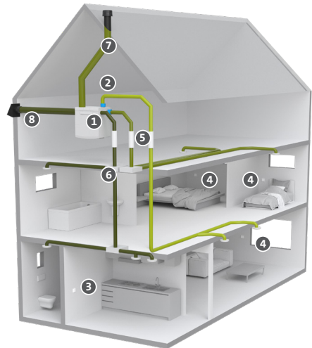
Overzicht ventilatie systeem HRC-EcoSmart/SmartComfort
