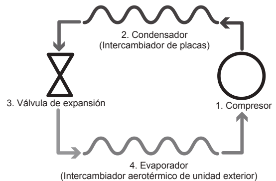
Esquema del sistema duo compacto
