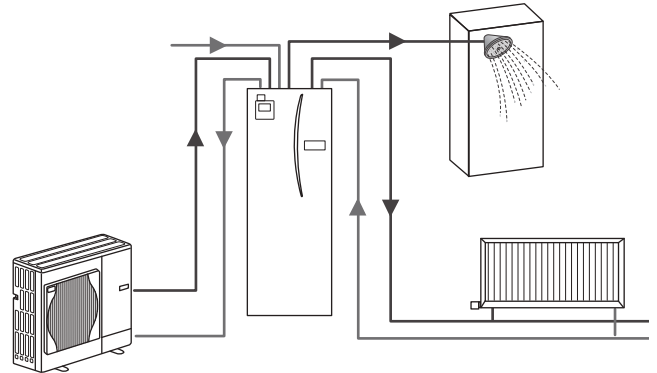
Pakettivaraajajärjestelmän kaavioesitys
