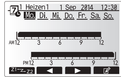
Vorschauenfenster
