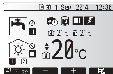
Startskjerm bilde
