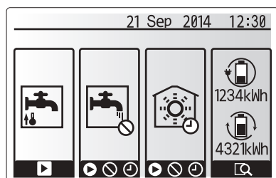
Alternativskjerm bilde
